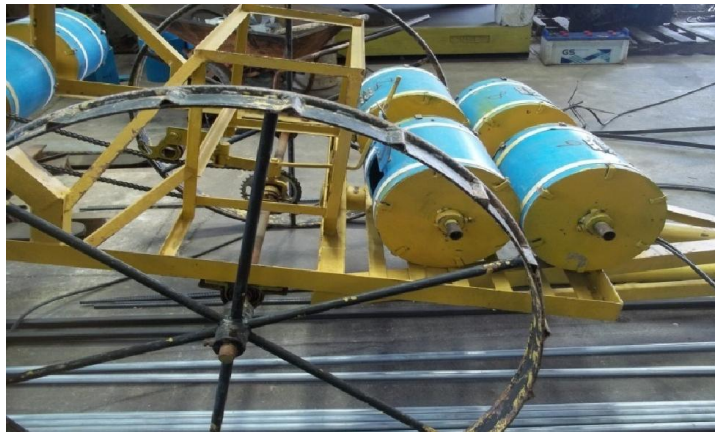
เครื่องหยอดเมล็ดพันธุ์ข้าว ขนาด กว้าง 1 เมตร ยาว 90 เซนติเมตร สูง 80 เซนติเมตร
