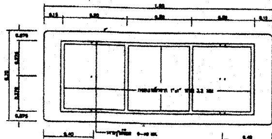
รายละเอียดการก่อสร้างฝาย
