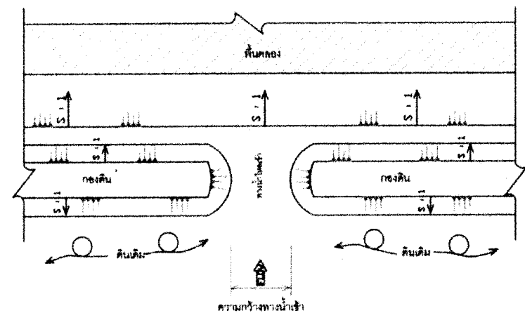
รูปแสดงการเว้นช่องทางน้ำเข้า
