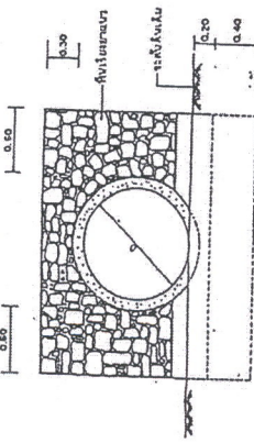
แบบ ข. กำแพงหัวท้อ ชนิดหินเรียงยาแนว
