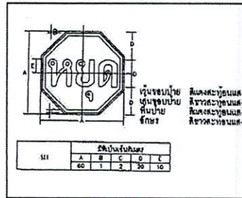
แบบป้ายจราจร (ป-๑๑) ประเภทป้ายบังคับ (บ-๑)
