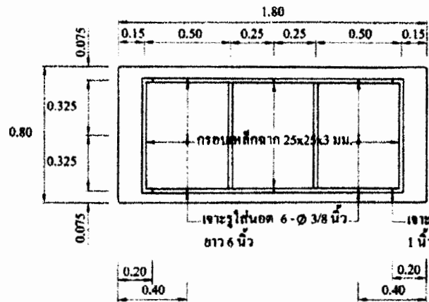
แสดงตำแหน่ง เจาะรูนอก มาตราส่วน 1 : 20
