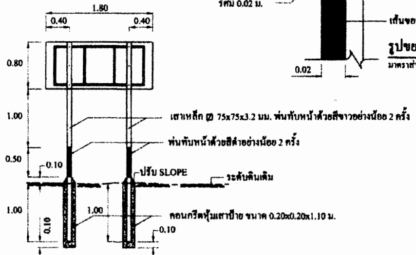
รายละเอียดการติดตั้งปาย มาตราส่วน 1 : 40
